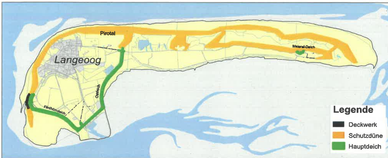
Abb. 2: Küstenschutzsystem auf Langeoog
