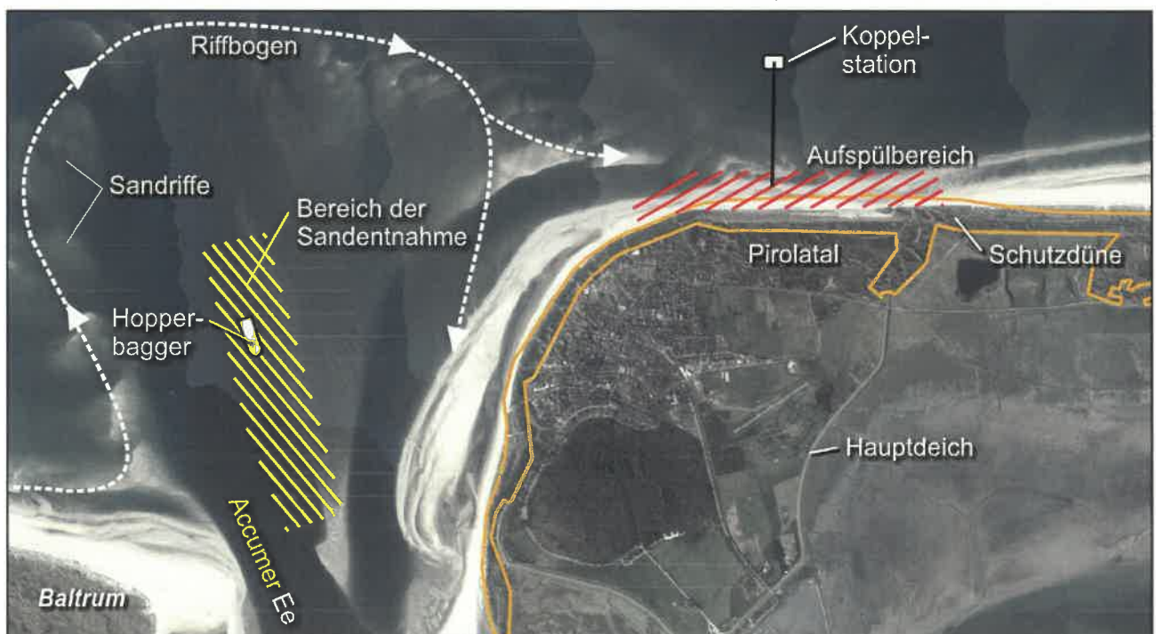
Abb. 1: Sandtransport und Übersichtsplan Strandaufspülung
