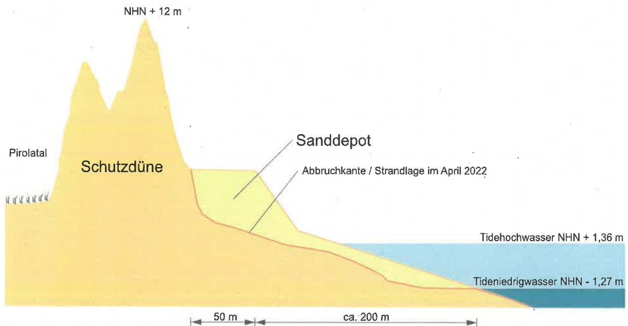
Abb. 3: Neues Strandprofil mit Sanddepot (überhöhte Darstellung)
